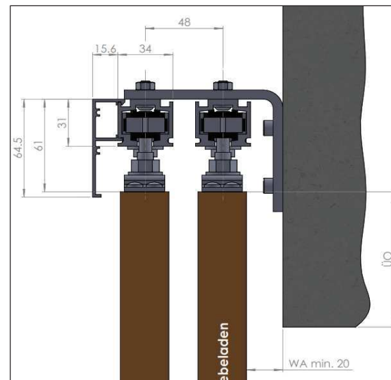
☐ Laufschiene Bügelmontage so2
