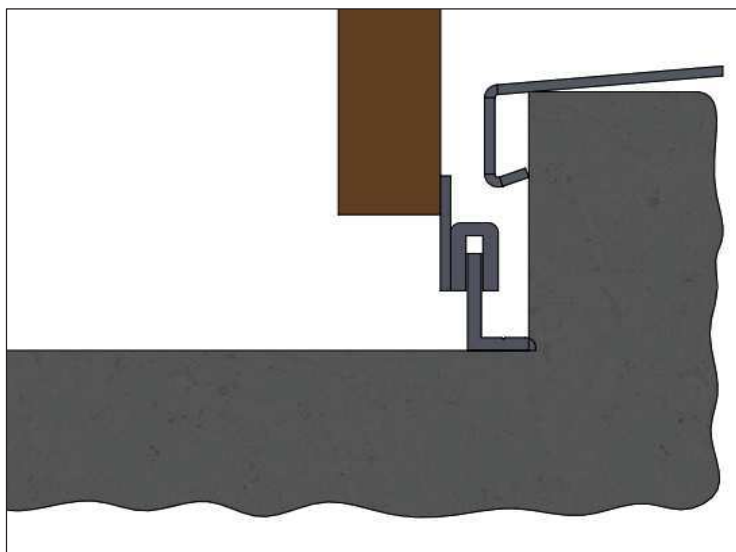
□ Montagesituation SU2 mit AK-Gleiter
