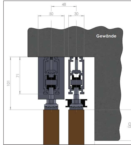
☐ Laufschiene Bügelmontage so2
