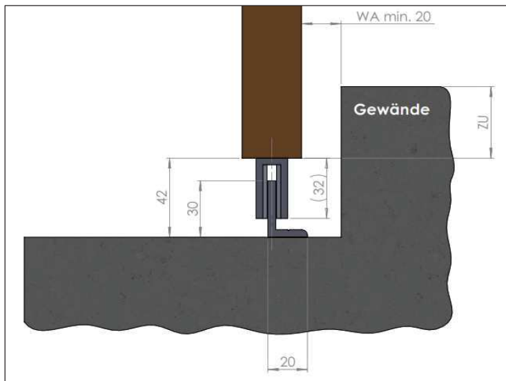
□ Montagesituation SU2 mit AK-Gleiter
