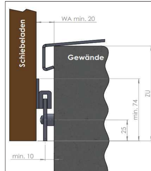
□ Montagesituation SU24 mit AK-Gleiter
