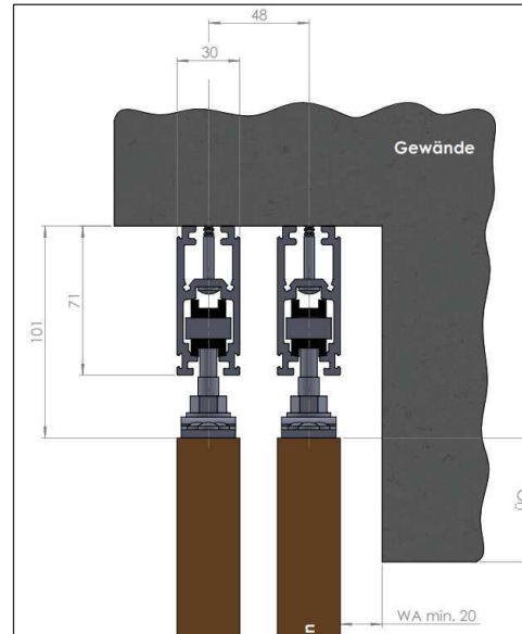
□ Laufschiene Bügelmontage so2
