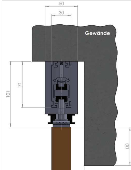
☐ Laufschiene Bügelmontage so2
