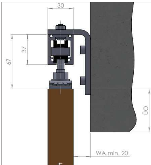
□ Laufschiene Bügelmontage so2
