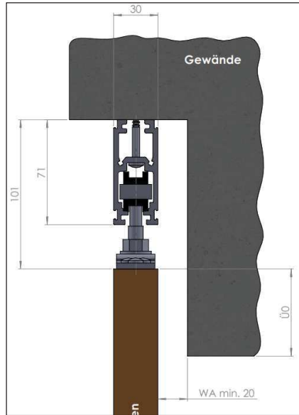
□ Laufschiene Bügelmontage so2
