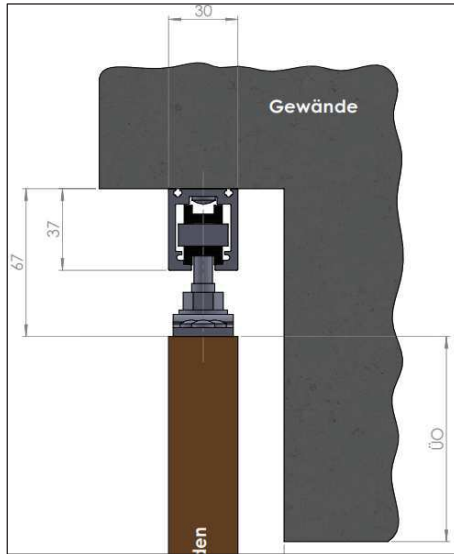
□ Laufschiene Bügelmontage so2
