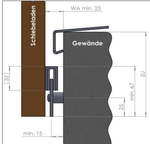
□ Montagesituation SU8 H-Gleiter
