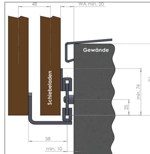
□ Montagesituation SU24 mit AK-Gleiter
