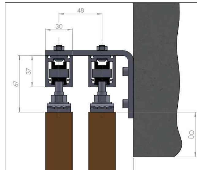
□ Laufschiene Bügelmontage so2
