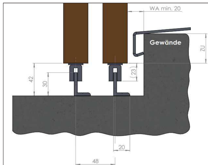
□ Montagesituation SU1 AK-Gleiter
