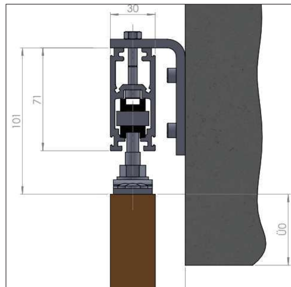
□ Laufschiene Bügelmontage so2
